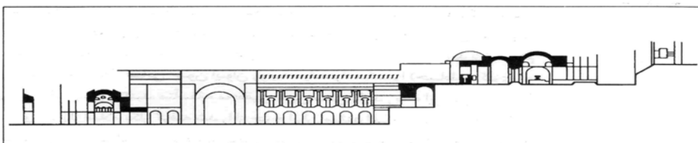
آرسن کوه خواجه، برش طولی (از کتاب میراثوری پارتها)
