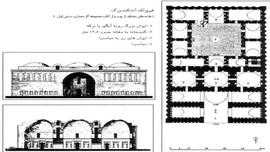
آتشکده فیروزآباد، نمای اصلی آتشکده فیروزآباد، برش از سه کنیذخانه.
